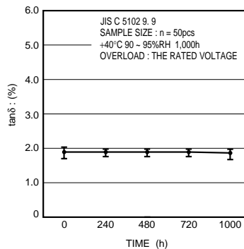
Fig.29 tanδ
