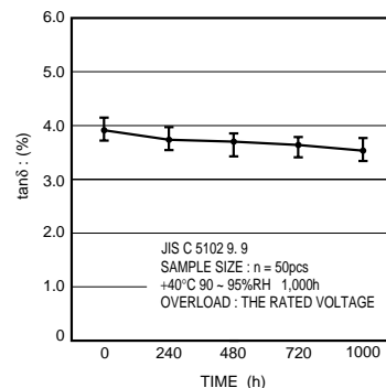
Fig.32 tanδ
