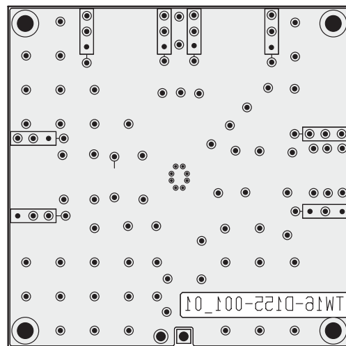
Bottom Layer
