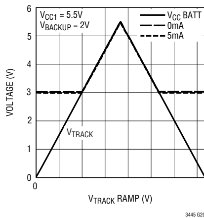
V_{CC BATT} vs V_{TRACK}
