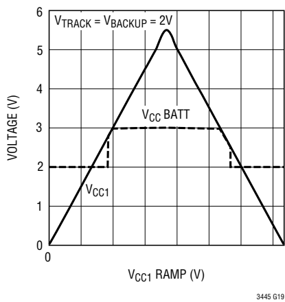
V_{CC BATT} vs V_{CC1}
