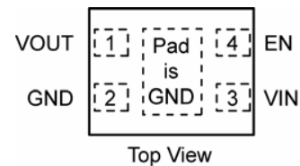
1.2x1.6 mm Thin MLF ® (MT)
